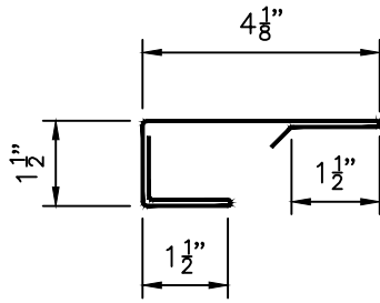
Optional Jamb Trim F484 Top View
